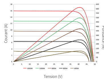
Courbes courant-tension et puissance-tension (615W)
